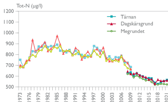
Figur 3. Medelhalt av totalkväve i ytvatten (0,5 m) vid Tärnan (Värmlandssjön), Dagskärsgrund (Skaraborgssjön) och Megrundet (Dalbosjön) 1973-2021. OBS! Skalan börjar på 500 µg/l, vilket förstärker skillnaden i resultat från de två olika analysmetoderna "Summakväve" och "TNb" (se Årsskrift 2009 för mer information om analysmetoderna).
