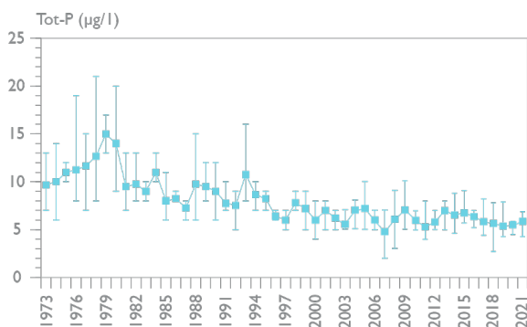
Figur 4. Medel-, min- och maxhalt av totalfosfor i ytvatten (0,5 m) vid Tärnan (Värmlandssjön) 1973-2021.
