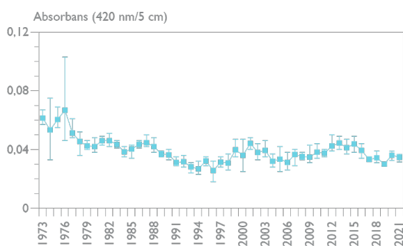
Figur 10. Medel-, min- och maxvärden av vattenfärgen (mätt som vattnets absorbans i 5-cm:s kyvett vid 420 nm) i ytvatten (0,5 m) vid Tärnan (Värmlandssjön) 1973-2021.
