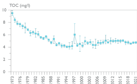
Figur 6. Medel-, min- och maxhalt av organiskt material (TOC) i ytvatten (0,5 m) vid Tärnan (Värmlandssjön) 1973-2021.
