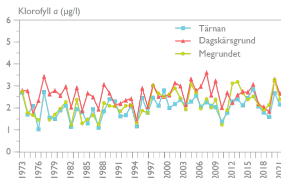
Figur 13. Medelhalt av klorofyll a i ytvatten (0-8 m) vid Tärnan (Värmlandssjön), Dagskärsgrund (Skaraborgssjön) och Megrundet (Dalbosjön) 1973-2021.
