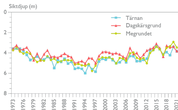
Figur 9. Medelsiktdjup vid Tärnan (Värmlandssjön), Dagskärsgrund (Skaraborgssjön) och Megrundet (Dalbosjön) 1973-2021.
