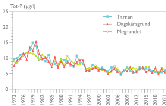
Figur 5. Medelhalt av totalfosfor i ytvatten (0,5 m) vid Tärnan (Värmlandssjön), Dagskärsgrund (Skaraborgssjön) och Megrundet (Dalbosjön) 1973-2021.
