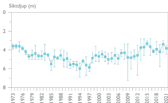
Figur 8. Medel-, min- och maxsiktdjup vid Tärnan (Värmlandssjön) 1973-2021.
