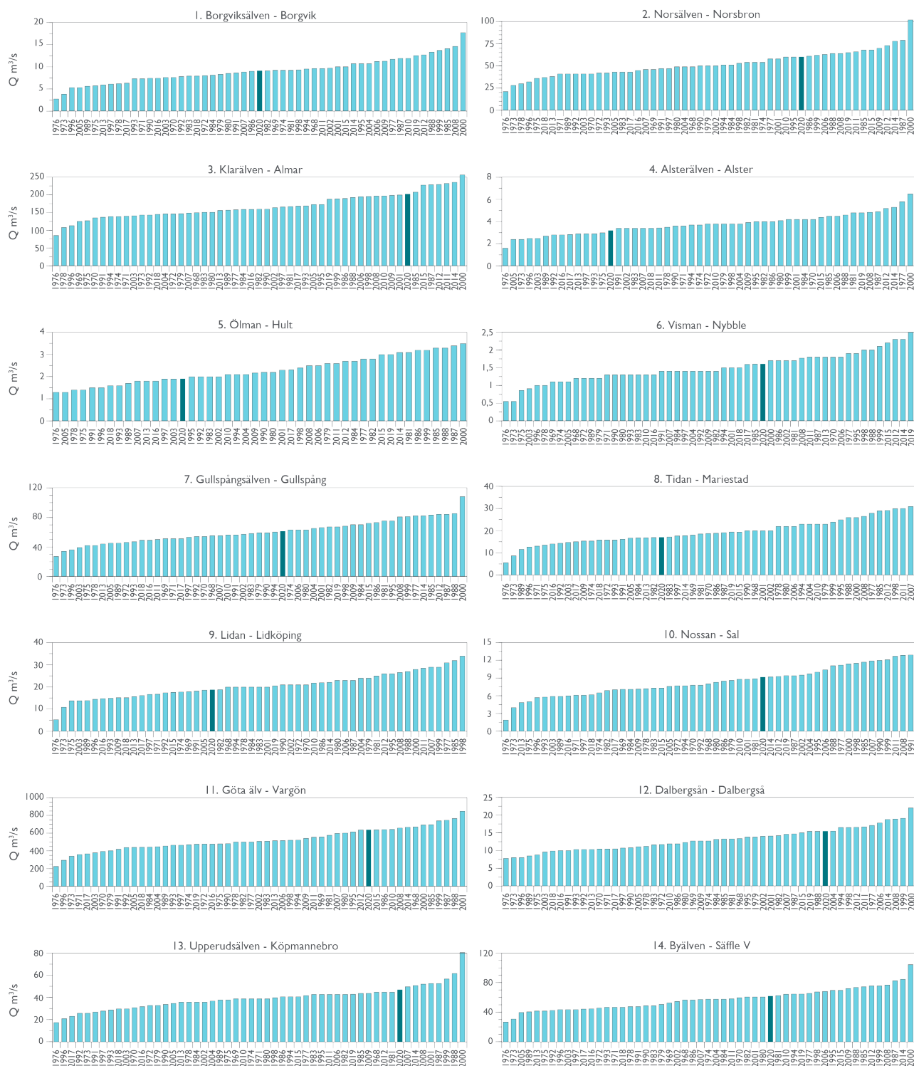
Figur 3. Årsmedelvattenföring i Vänerns tillflöden och utlopp rangordnade från det lägsta till det högsta registrerade värdet för respektive vattendrag. Mörkblå stapel markerar år 2020.
