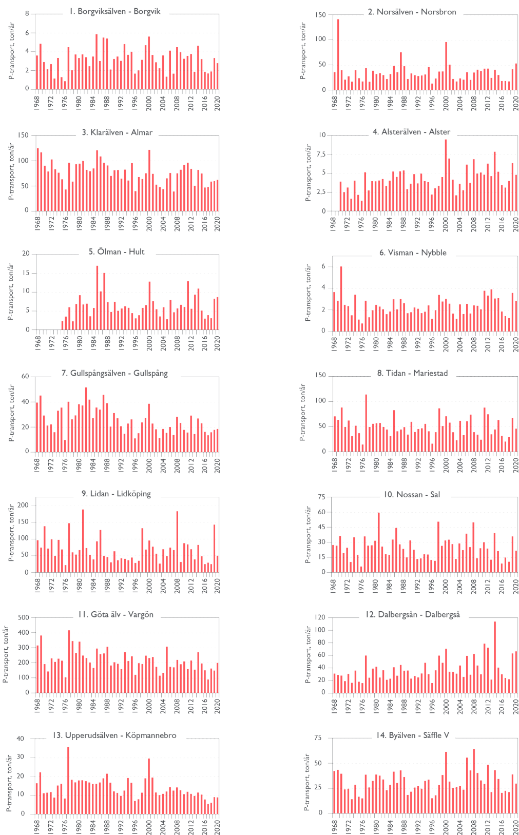
Figur 6. Årstransport av fosfor via Vänerns tillflöden och utlopp 1968–2020. OBS! De olika diagrammen har olika skalor. Haltuppgifter för Tidan, Lidan och Nossan fr o m 2008, samt Dalbergsån fr o m 2013 kommer från den samordnade recipientkontrollen.
