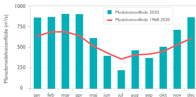
Figur 2. Månadsmedelvattenflöden i Göta älv vid Vargön för 2020 och perioden 1968–2020.
