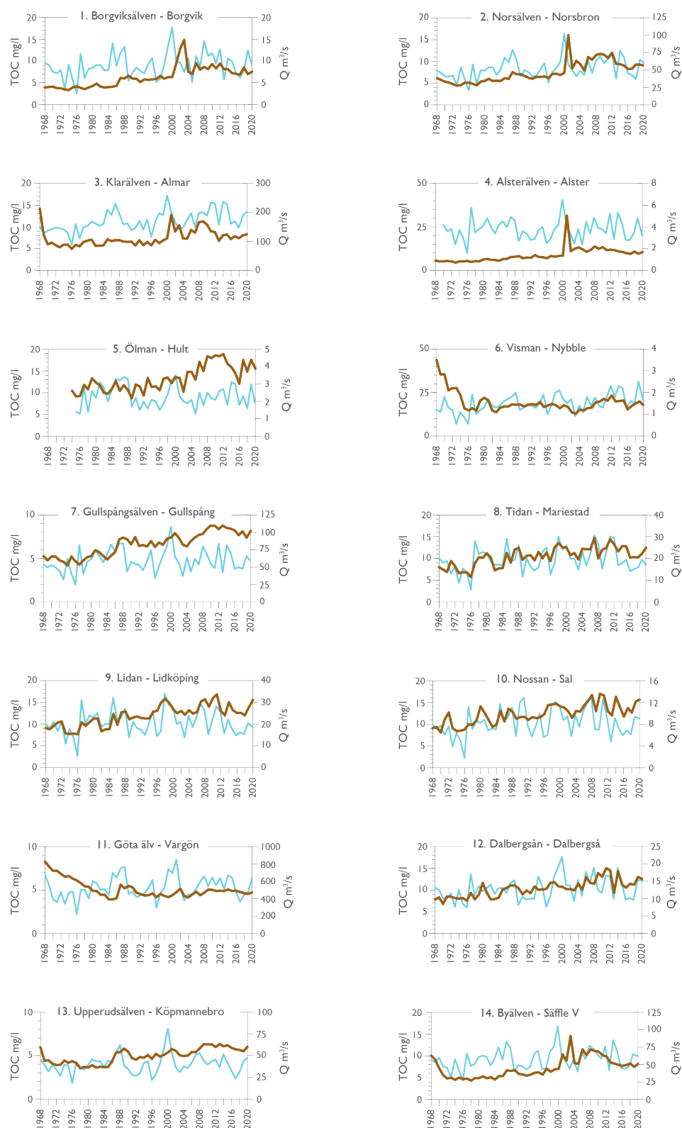
Figur 9. Tidsutvecklingen för organiskt material (TOC) (brun linje), samt vattenföring (ljusblå linje) i Vänerns tillflöden och utlopp 1968–2020. Skalorna har anpassats så att båda kurvorna ska ligga så nära varandra som möjligt för att kunna avgöra graden av samvariation. Haltuppgifter för Tidan, Lidan och Nossan fr o m 2008, samt Dalbergsån fr o m 2013 kommer från den samordnade recipientkontrollen. TOC för perioden fram till och med 1986 har beräknats utifrån vattnets kemiska syrgasförbrukning ( COD_{Mn} = 1,24 \cdot TOC ).
