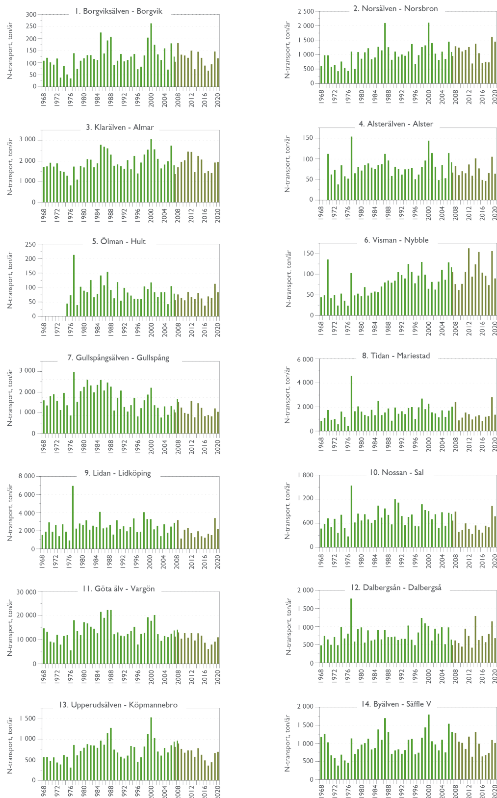
Figur 5. Årstransport av kväve via Vänerns tillflöden och utlopp 1968–2020. OBS! De olika diagrammen har olika skalor. Fram till 2008 är totalkvävet analyserat som "summakväve" (gröna staplar). De mörkgröna staplarna därefter anger totalkvävet som "TNb", förutom för data från den samordnade recipientkontrollen för Tidan, Lidan och Nossan där dessa avser "persulfatuppslutet" kväve. För Dalbergsån avses "TNb" 2008-2012 och därefter "persulfatuppslutet" kväve.
