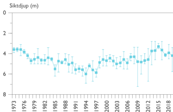
Figur 8. Medel-, min- och maxsiktdjup vid Tärnan (Värmlandssjön) 1973-2019.
