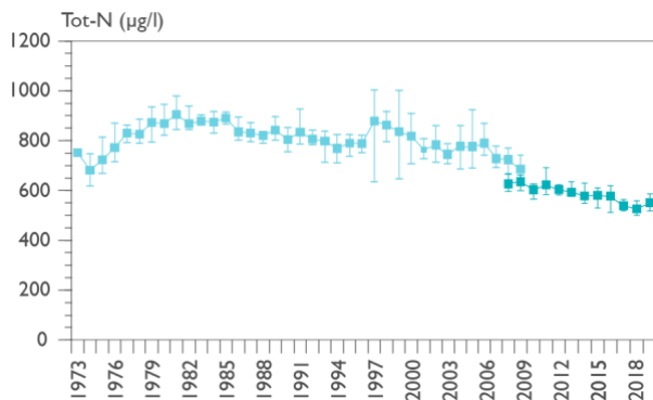
Figur 2. Medel-, min- och maxhalt av totalkväve i ytvatten (0,5 m) vid Tärnan (Värmlandssjön) 1973-2019. OBS! Totalkvävehalten visas som "Summakväve" (summan av Kjeldahlkväve och nitrit+nitratkväve) till och med 2009 och som "TNb" (totalhalten mätt som kväveoxider efter förbränning) från och med 2008. Summakvävet illustreras med ljusblå punkter och linjer, TNb med mörkblå.
