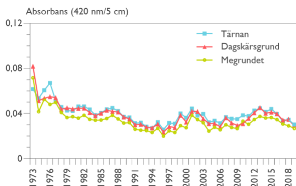
Figur 11. Medelvattenfärgen (mätt som vattnets absorbans i 5-cm:s kyvett vid 420 nm) vid Tärnan (Värmlandssjön), Dagskärsgrund (Skaraborgssjön) och Megrundet (Dalbosjön) 1973-2019.
