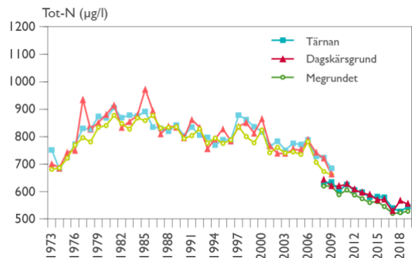
Figur 3. Medelhalt av totalkväve i ytvatten (0,5 m) vid Tärnan (Värmlandssjön), Dagskärsgrund (Skaraborgssjön) och Megrundet (Dalbosjön) 1973-2019. OBS! Skalan börjar på 500 µg/l, vilket förstärker skillnaden i resultat från de två olika analysmetoderna "Summakväve" och "TNb" (se Årsskrift 2009 för mer information om analysmetoderna).
