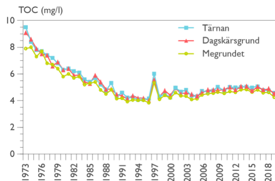
Figur 7. Medelhalt av organiskt material (TOC) i ytvatten (0,5 m) vid Tärnan (Värmlandssjön), Dagskärsgrund (Skaraborgssjön) och Megrundet (Dalbosjön) 1973-2019.
