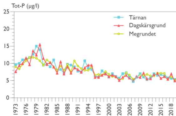
Figur 5. Medelhalt av totalfosfor i ytvatten (0,5 m) vid Tärnan (Värmlandssjön), Dagskärsgrund (Skaraborgssjön) och Megrundet (Dalbosjön) 1973-2019.
