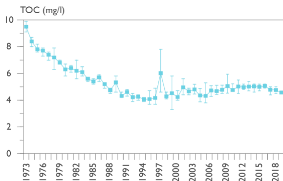
Figur 6. Medel-, min- och maxhalt av organiskt material (TOC) i ytvatten (0,5 m) vid Tärnan (Värmlandssjön) 1973-2019.
