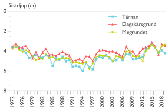
Figur 9. Medelsiktdjup vid Tärnan (Värmlandssjön), Dagskärsgrund (Skaraborgssjön) och Megrundet (Dalbosjön) 1973-2019.
