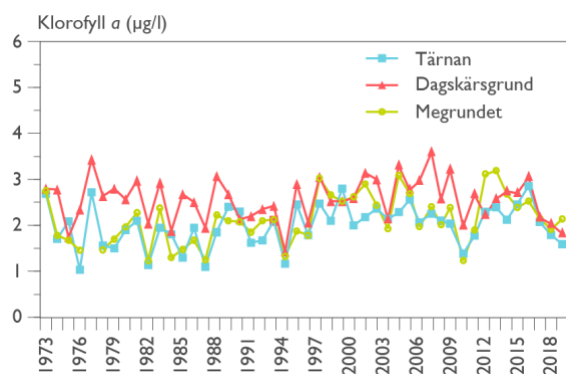
Figur 13. Medelhalt av klorofyll a i ytvatten (0-8 m) vid Tärnan (Värmlandssjön), Dagskärsgrund (Skaraborgssjön) och Megrundet (Dalbosjön) 1973-2019.
