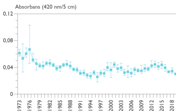
Figur 10. Medel-, min- och maxvärden av vattenfärgen (mätt som vattnets absorbans i 5-cm:s kyvett vid 420 nm) i ytvatten (0,5 m) vid Tärnan (Värmlandssjön) 1973-2019.
