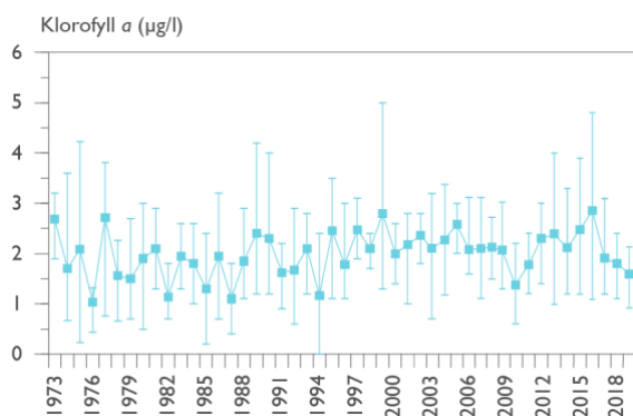
Figur 12. Medel-, min- och maxhalt av klorofyll a i ytvatten (0-8 m) vid Tärnan (Värmlandssjön) 1973-2019.
