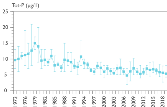
Figur 4. Medel-, min- och maxhalt av totalfosfor i ytvatten (0,5 m) vid Tärnan (Värmlandssjön) 1973-2019.
