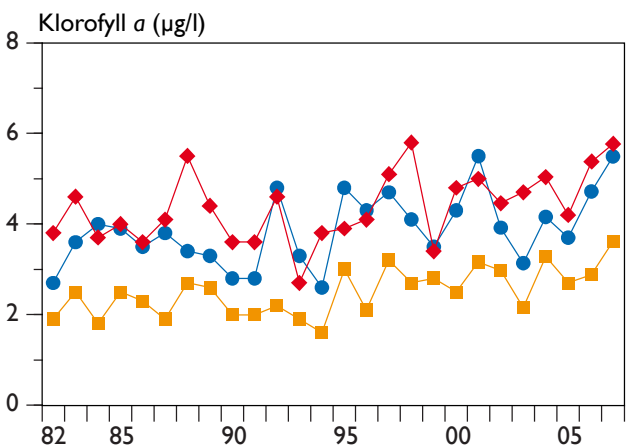
Figur 9. Klorofyllhalt i ytvatten (0,5 m) vid M1 och M2 i Mariestadsfjärden, samt vid Dagskärsgrund i Storvänern. Samtliga data är medelvärden för resp. provtagningssäsong 1982–2007. Symboler enligt figur 3.
