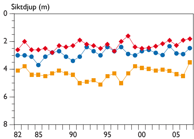
Figur 7. Siktdjupet vid M1 och M2 i Mariestadsfjärden, samt Dagskärsgrund i Storvänern. Samtliga data är medelvärden för resp. provtagningssäsong 1982–2007. Symboler enligt figur 3.
