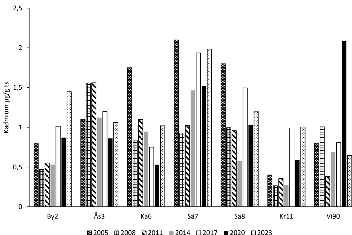
Figur 16. Medelhalt kadmium uttryckt som \mu\text{g/g ts} i abborrelever från lokalerna i norra Vänern under 2005–2023. Observera att halterna 2011–2017 är medelvärden hämtade från årsrapporter (Norborg Carlsson 2012, 2015, 2019) och att halterna 2005 är uppskattade från diagram i Grotell (2018). Lokalerna förkortas enligt: Byviken (By2), Ås fjorden (Ås3), Kattfjorden (Ka6), Hammarösjön (Sä7), Sätterholmsfjärden (Sä8), Varnumsviken (Kr11) samt Kolstrandsviken (Vi90).
