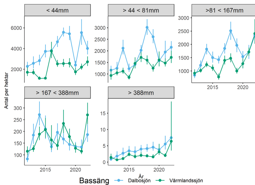
Figur 3. Antal fiskar per hektar (oavsett art) och år (2012-2022) för fem olika storlekklasser, <44 mm, 44 - 81 mm, 81 – 167 mm, 167 – 388 mm och > 388 mm (omräknade från ekostyrka). Värdena är medelvärden beräknade för Dalbosjön och Värmlandssjön, och spridningen (vertikala linjer) visar 95 % konfidensintervall, skattade med bootstrap.
